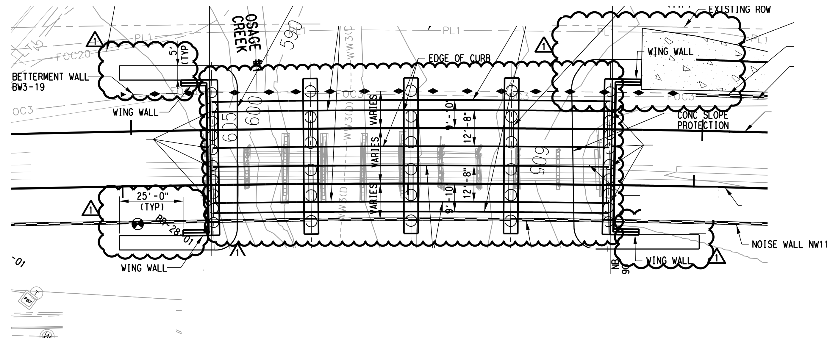
PLAN SCALE: 1" = 20'
